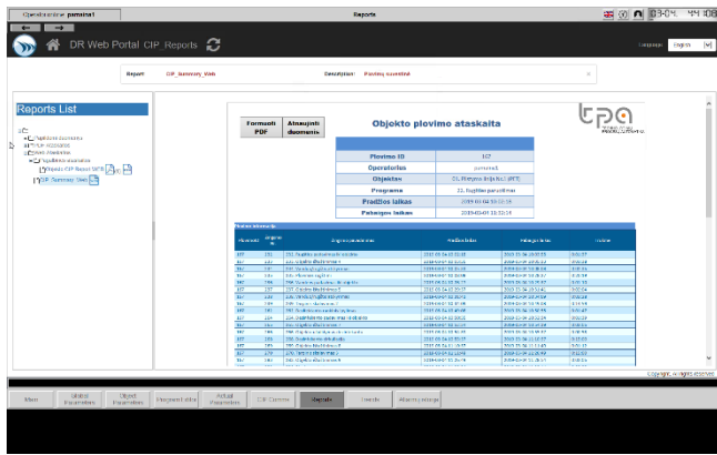
Рисунок 2 Детализированный Веб-отчёт выбранной последовательности CIP процедур.
